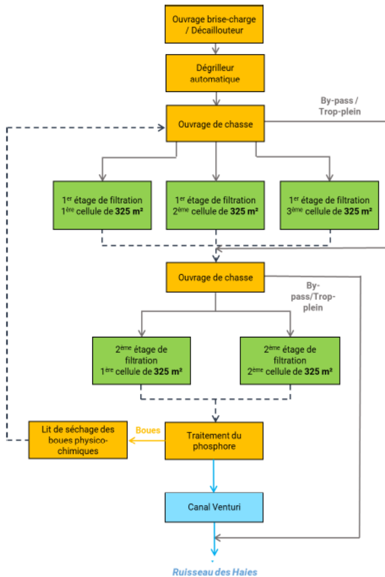
Figure 3 : Synoptique de la filière de traitement
